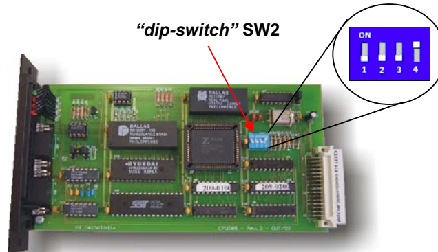
Figura - Localização da "dip-switch" de inicialização do módulo CPU209-Revisão2
