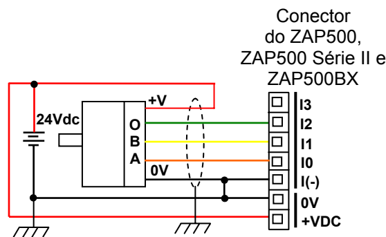
Figura – Esquema de ligação do encoder no ZAP500, ZAP500 Série II e ZAP500BX
