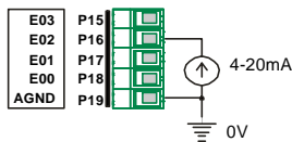
ZEM530 - Exemplo de conexão de entradas analógicas
