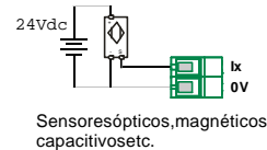
Exemplos de conexões das entradas digitais I8 a I11.
