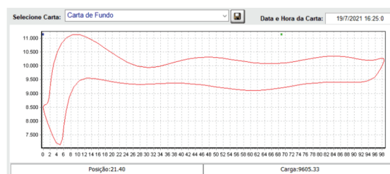
Carta dinamométrica de fundo
